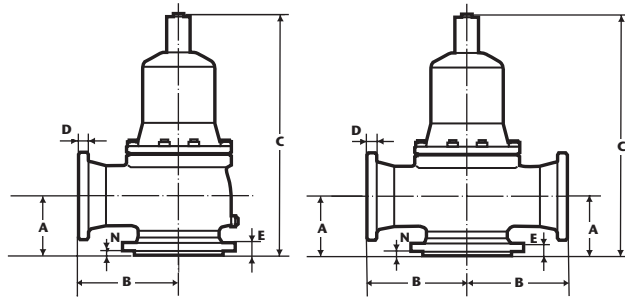
Orifice V
